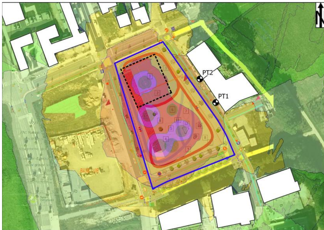
Figure 8 : Cathographie sonore - traitements de priorité 1
